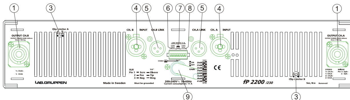
Figure 2 : Panneau arrière
